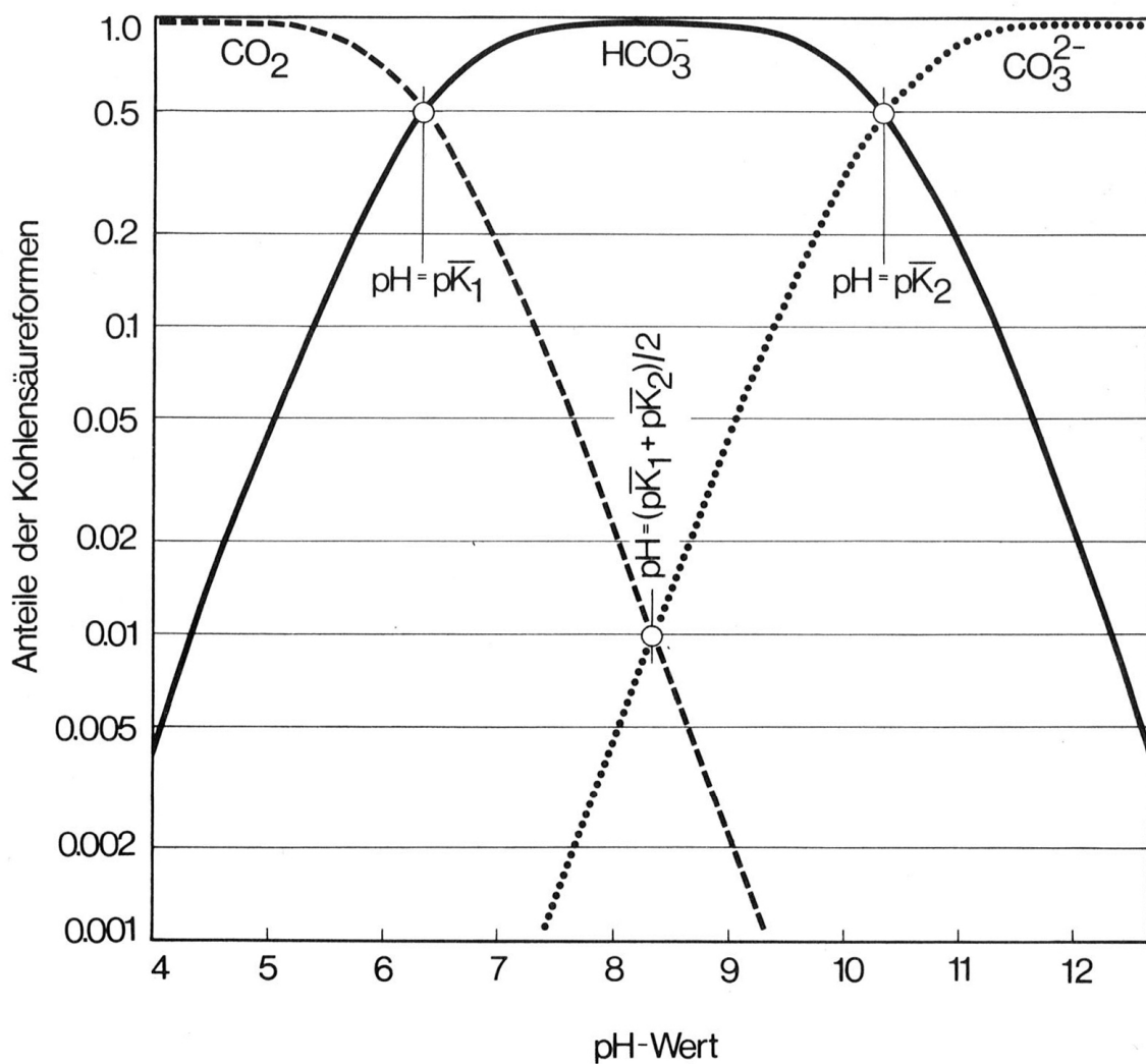
Abbildung 4.2 Anteile der Kohlensäureformen an der Gesamtkohlensäure in Abhängigkeit vom pH-Wert für \vartheta = 25\text{ }^\circ\text{C} , \mu = 0\text{ mol/l}
