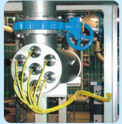
UV-Anlagen
